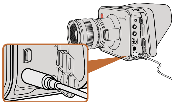
Для зарядки встроенной батареи и питания камеры используется прилагаемый сетевой адаптер
