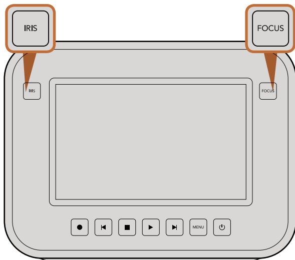
Cinema Camera와 Production Camera 4K EF 모델에서는 IRIS 버튼 또는 트랜스포트 컨트롤을 사용하여 조리개를 조절할 수 있습니다. FOCUS 버튼을 누르면 포커스 피킹이 실행됩니다. EF 마운트 모델에서 호환 렌즈를 사용할 시, FOCUS 버튼을 누르면 자동 초점 기능을 실행합니다.
