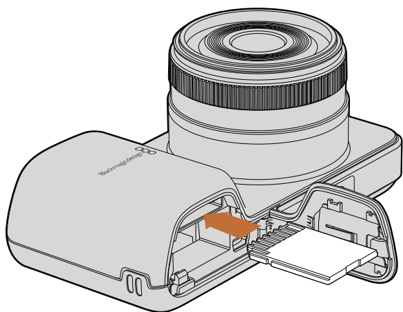
Insertión de una tarjeta SD (Pocket Cinema Camera)
