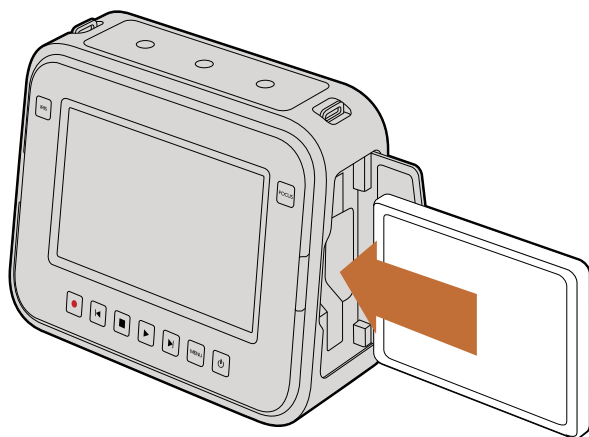
Insertión de un dispositivo SSD (Cinema Camera / Production Camera 4K)
